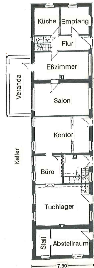
ERDGESCHOß
