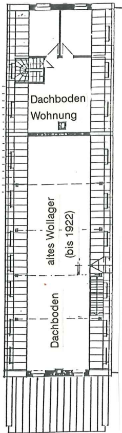
2. OBERGESCHOß
