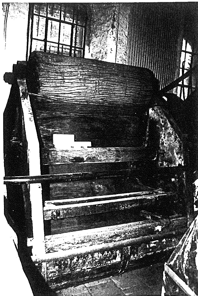
Abb. 10. Die Objekte in der Naßappretur wurden im Übernahmestand erhalten. Das bedeutete neben der Erhaltung von Gebrauchs- und Stilllegungsspuren auch die Konservierung der Verfallsspuren, die nach 1961 bis zum Beginn der Inventarsanierung 1996/97 aufgetreten waren.
