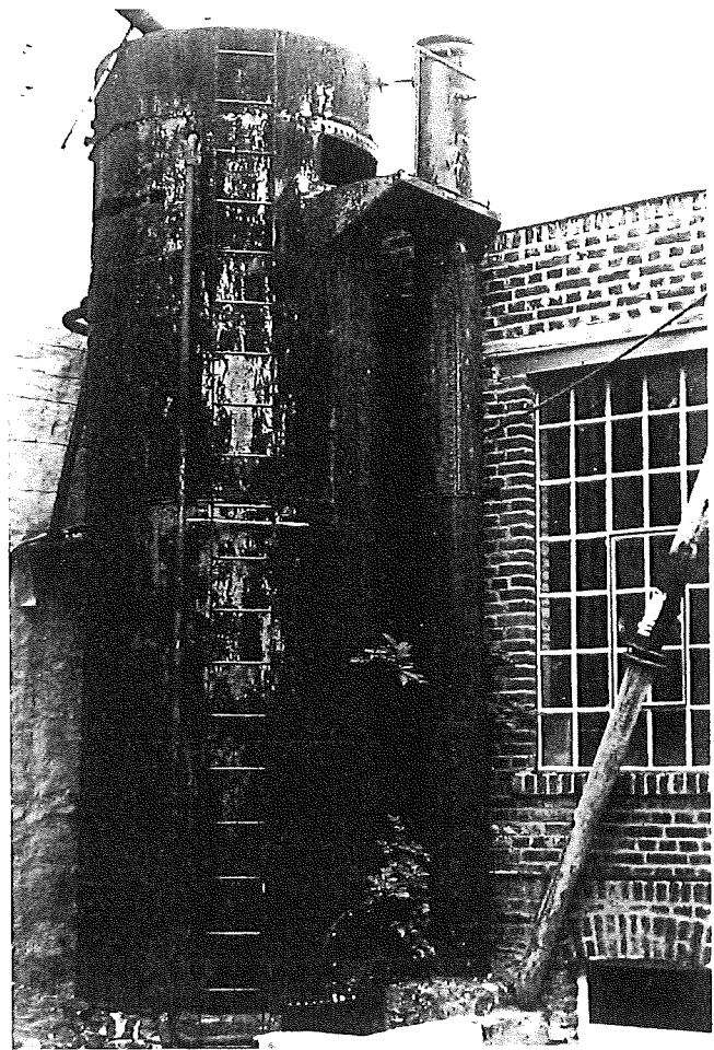
Abb. 11. Der Wasseraufbereitungstank im Fabrikhof: Seine ursprüngliche schwarze Beschichtung war durch jahrzehntelange Freilandbewitterung stark abgewittert.
